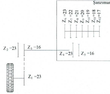
Şekil 1. Ekici Ünite Hareket İletimi
