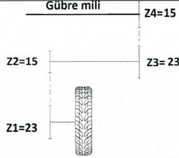
Şekil 2. Gübre Atıcı Hareket İletimi
