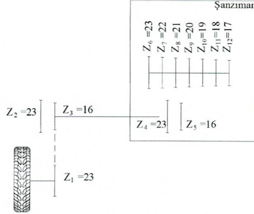
Şekil 1. Ekici Ünite Hareket İletimi
