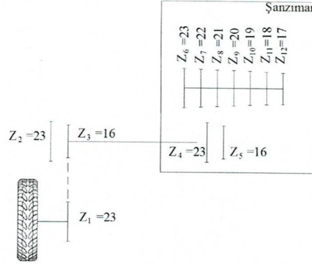
Şekil 1. Ekici Ünite Hareket İletimi
