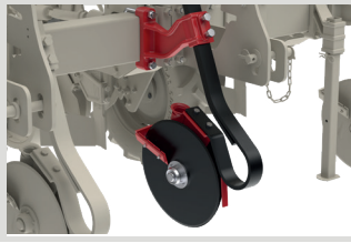
Çift Diskli Gübre Atıcı
