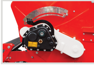
Ayarlanabilir Şanzıman
