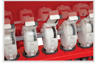
Her Türlü Tohumu Atabilen Tohum ve Gübre Gözleri
