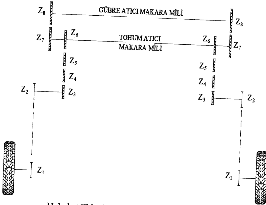
Hububat Ekim Makinesi Hareket İletim Şeması
